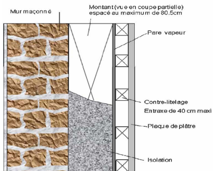
Figure 2 : Mur maçonné – isolation intérieure derrière un pare-vapeur
